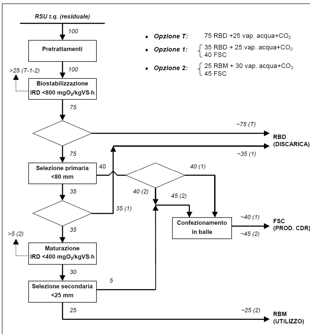
Figura 6.27: diagramma a blocchi del Decreto Commissariale 296/02
