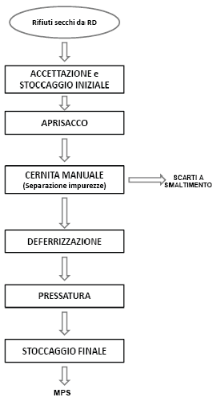
Figura 6. Diagramma di flusso tipico dei centri di selezione rifiuti secchi da RD presenti in Puglia
