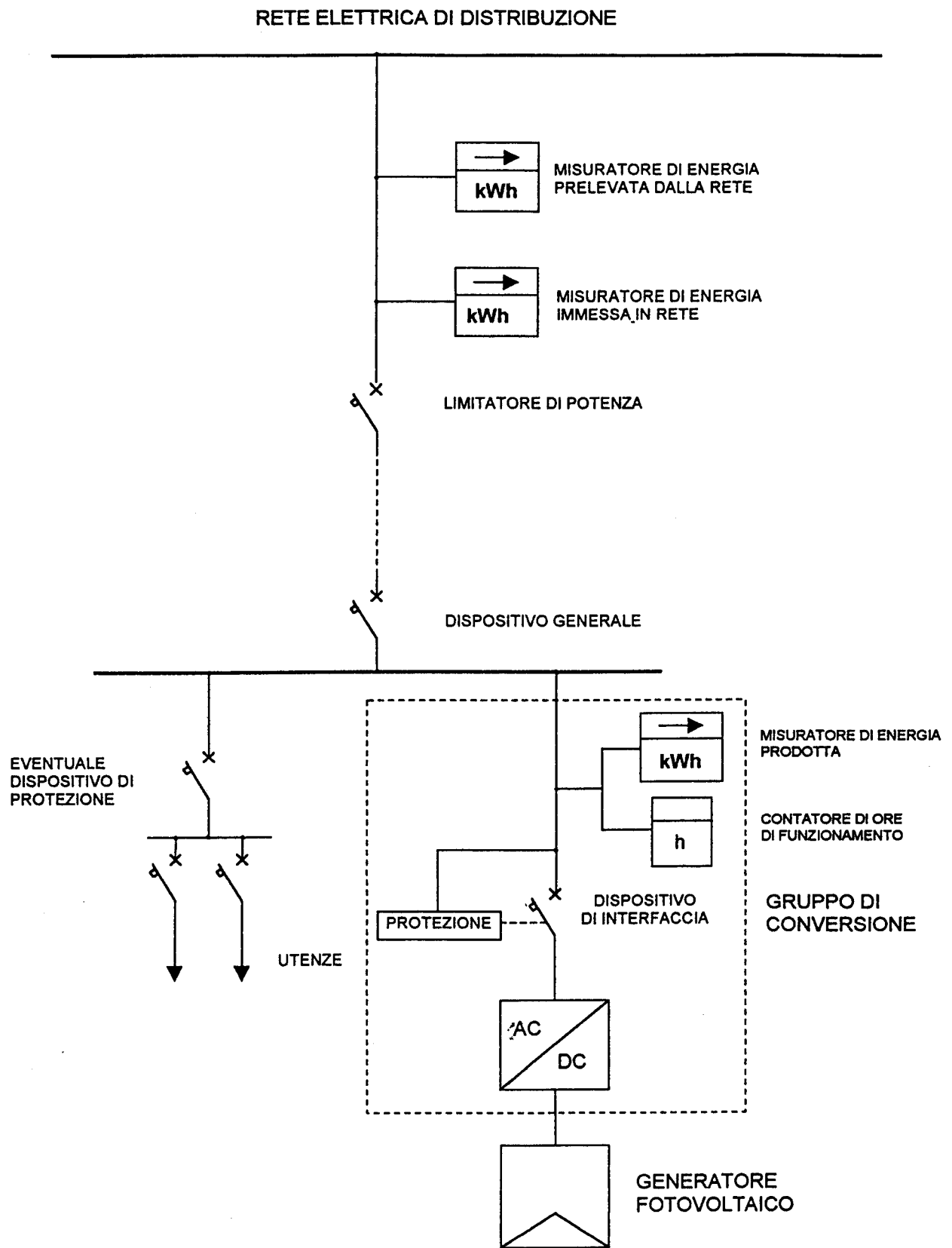
Figura 1: schema tipico di collegamento dell'impianto fotovoltaico alla rete elettrica di distribuzione
