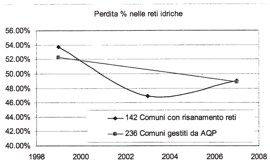
Figura 16: Sovrapposizione andamenti delle perdite
