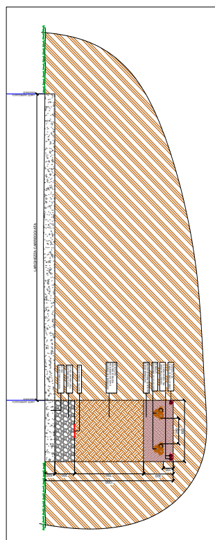
PARTICOLARE - SEZIONE A-B
