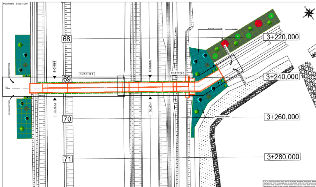
Stralcio tavola PC5.1 Opere a verde – sottopasso faunistico
