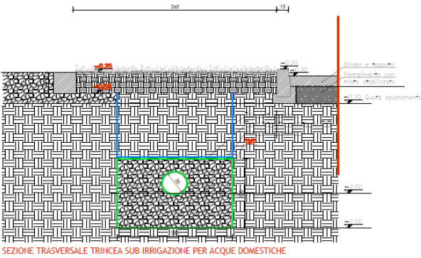
Figura 38: trincea drenante
