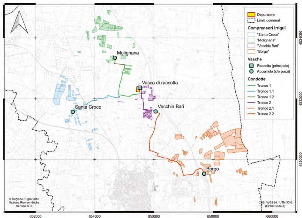
Figura 2: layout della rete, ubicazione dei compensatori irrigui
