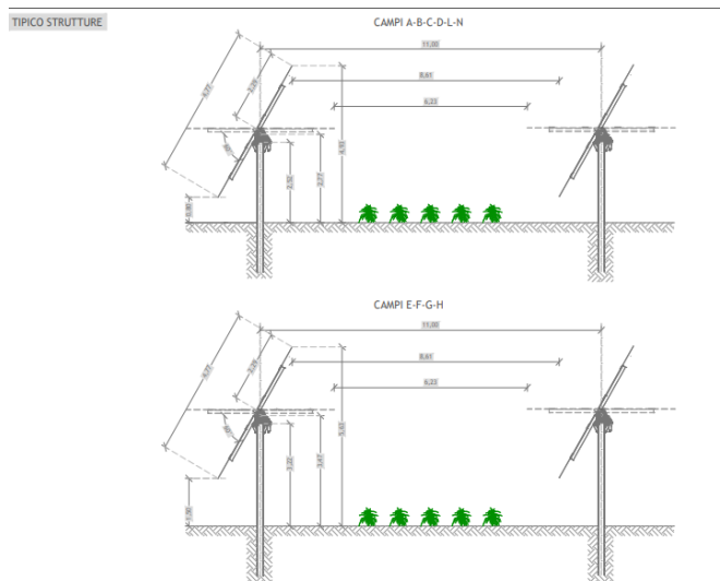
Figura 6 – Particolare strutture di progetto
