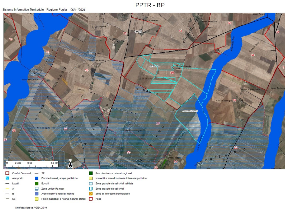
Figura 4: stralcio PPTR con individuazione catastale dell'impianto
