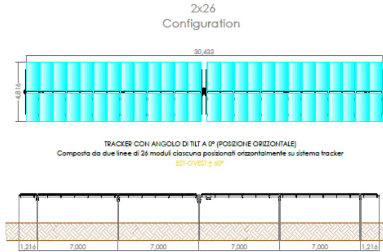
Figura 3: particolari strutture tracker
