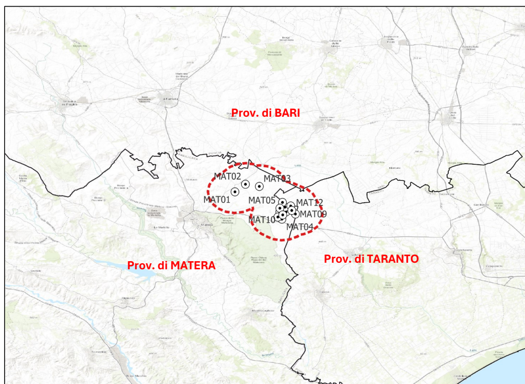
Fig. 1 - Ubicazione degli aerogeneratori in Basilicata, al confine con la Puglia.
