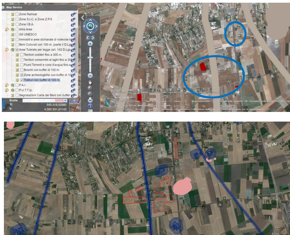
Fig. 1 - Area dell'impianto con buffer di 500 m rispetto a beni sottoposti a tutela (PPTR)
