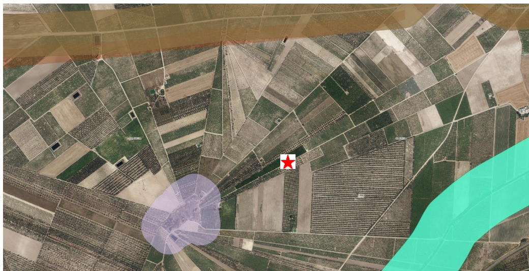
Fig. 6 - Particolare dell'impianto rispetto alle aree non idonee ex RR 24/2010 (aerogeneratore WTG 05 indicato con una stella rossa)
