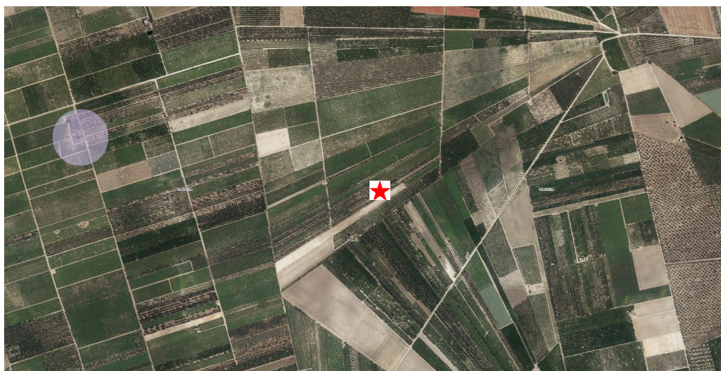
Fig. 7 - Particolare dell'impianto rispetto alle aree non idonee ex RR 24/2010 (aerogeneratore WTG 06 indicato con una stella rossa)
