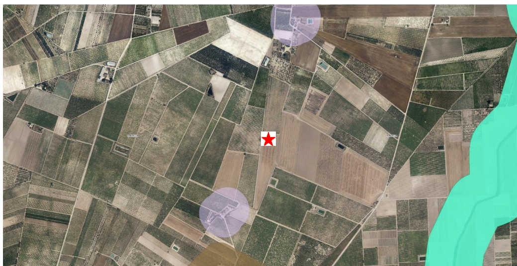
Fig. 5 - Particolare dell'impianto rispetto alle aree non idonee ex RR 24/2010 (aerogeneratore WTG 04 indicato con una stella rossa)
