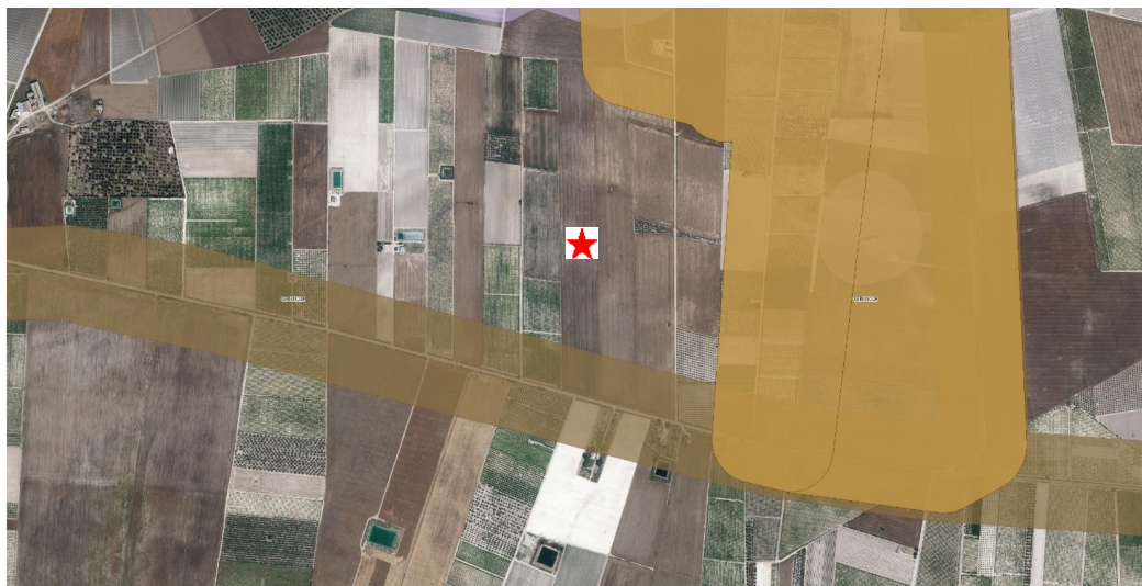
Fig. 4 - Particolare dell'impianto rispetto alle aree non idonee ex RR 24/2010 (aerogeneratore WTG 03 indicato con una stella rossa)
