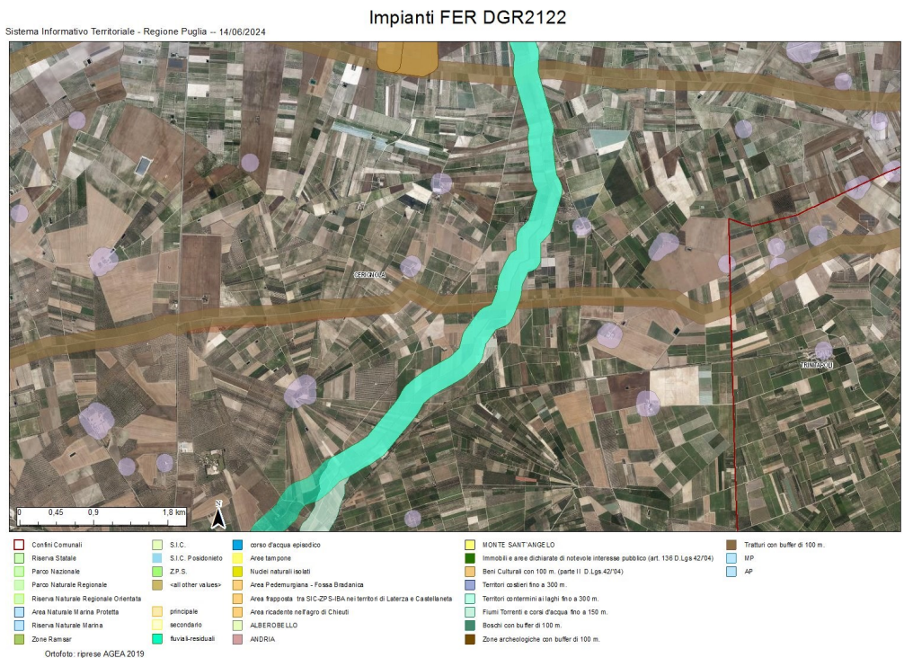
Fig. 2 - Ubicazione dell'impianto rispetto alle aree non idonee ex RR 24/2010 (gli 11 aerogeneratori sono indicati con una stella rossa)
