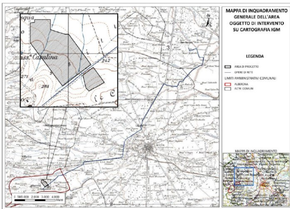
Figura 1: inquadramento del progetto su IGM (tavola progettuale)
