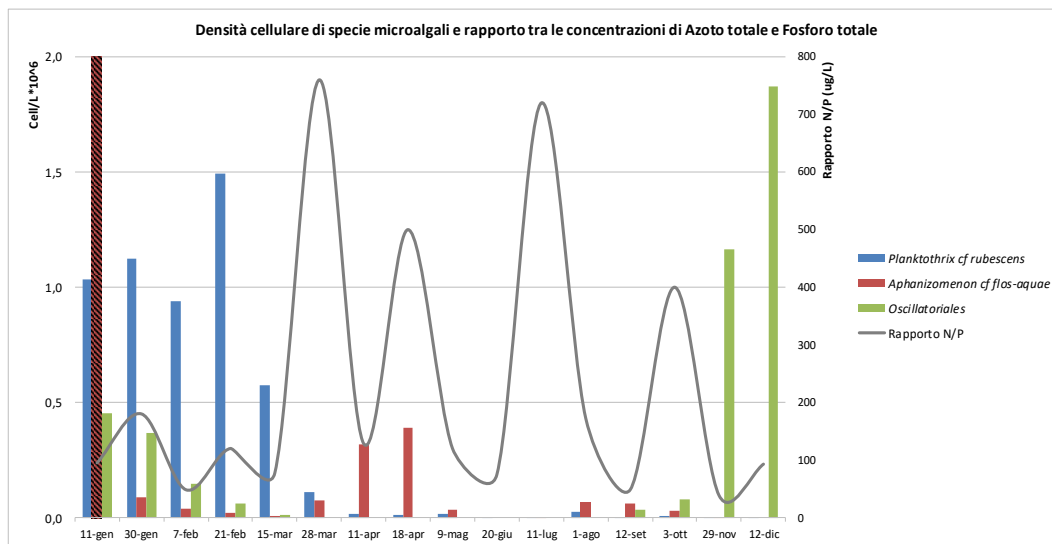
Densità cellulare delle specie microalgali potenzialmente tossiche rinvenute in superficie nella stazione di campionamento "Opera di presa". Andamento temporale del Rapporto N/P - Azoto totale su Fosforo totale, misurati nella medesima stazione di campionamento.
