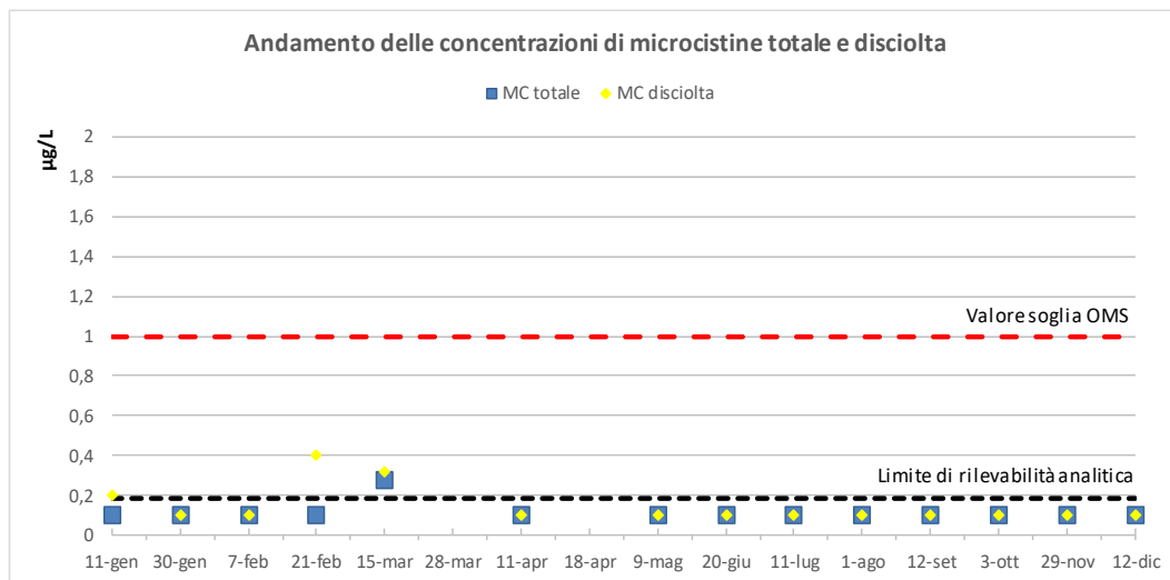
Concentrazione di microcistine disciolte e totali nell'Invaso di Occhito - Annualità 2023
