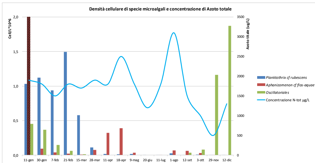
Densità cellulare delle specie microalgali potenzialmente tossiche rinvenute in superficie nella stazione di campionamento "Opera di presa". Andamento temporale dell'Azoto totale misurato nella medesima stazione di campionamento.
