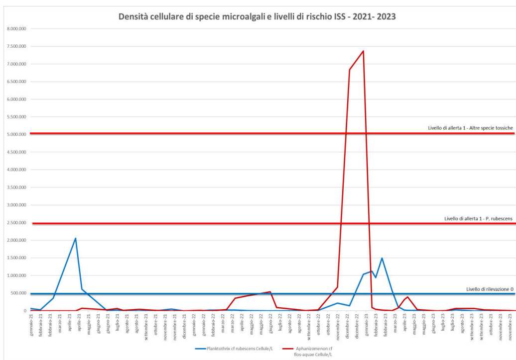
Densità cellulare delle specie microalgali potenzialmente tossiche P. rubescens e A. flos-aquae rinvenute in superficie nella stazione di campionamento “Opera di presa” nel triennio 2021-2023.
