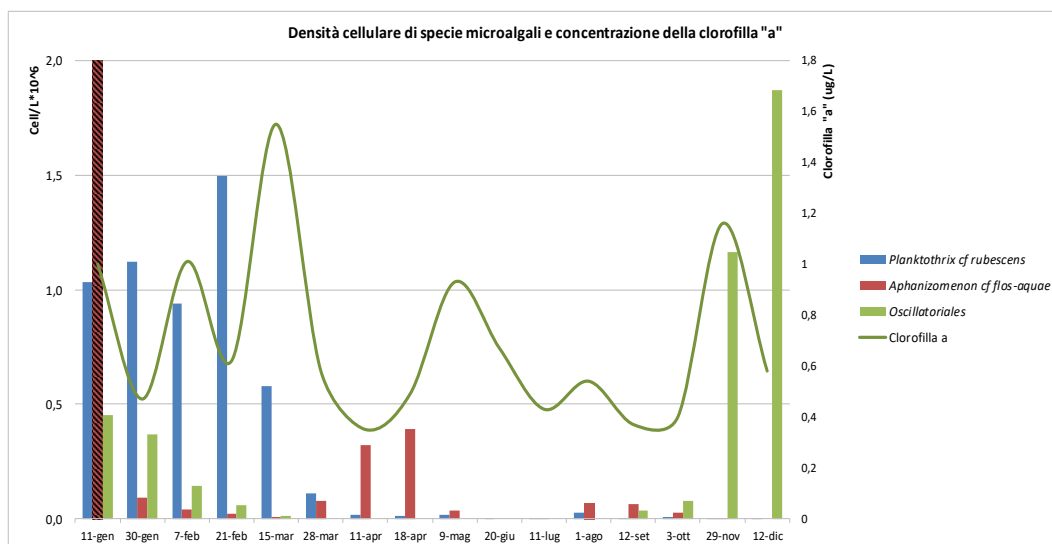
Densità cellulare delle specie microalgali potenzialmente tossiche rinvenute in superficie nella stazione di campionamento "Opera di presa". Andamento temporale della concentrazione di Clorofilla "a" misurata in superficie nella medesima stazione di campionamento.
