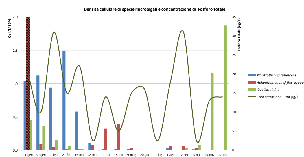
Densità cellulare delle specie microalgali potenzialmente tossiche rinvenute in superficie nella stazione di campionamento "Opera di presa". Andamento temporale del Fosforo totale misurato nella medesima stazione di campionamento.
