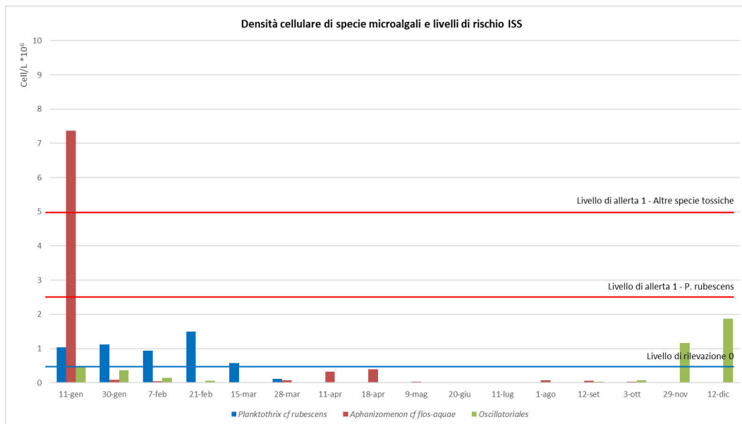
Densità cellulare delle specie microalgali nell'Invaso di Occhito - Annualità 2023 e livelli di rischio definiti dall'ISS
