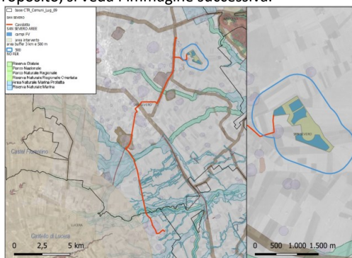
Figura 6 – Inquadramento su Aree non idonee F.E.R. e buffer di m. 500.
