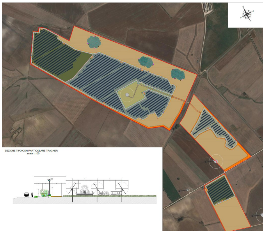
Figura 3: area effettiva dell'impianto fotovoltaico
