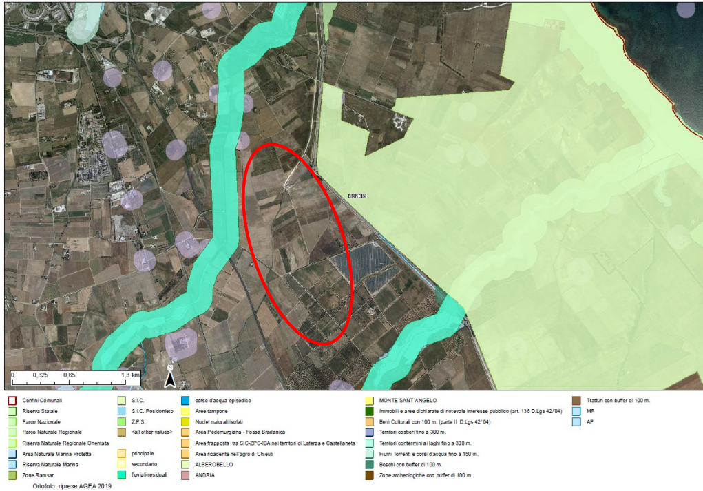
Fig. 1 - Ubicazione dell'impianto rispetto alle aree non idonee ex RR 24/2010
