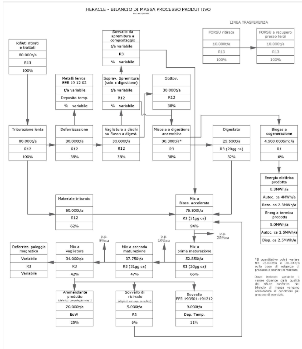
Figura 8: schema di flusso e bilancio di massa
