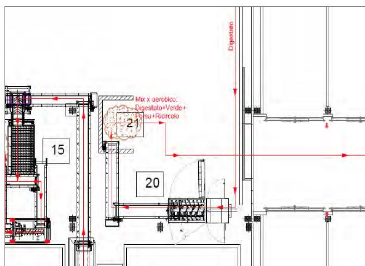
Figura 20: sezione miscelazione
