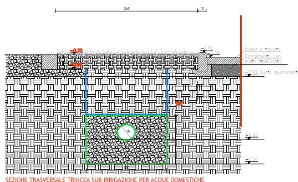
Figura 34: trincea drenante
