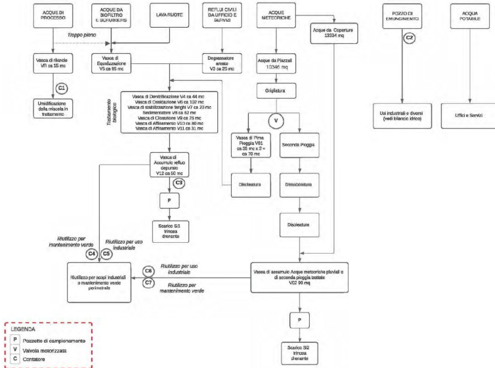
Figura 30: Schema di flusso gestione acque di stabilimento nella situazione attuale
