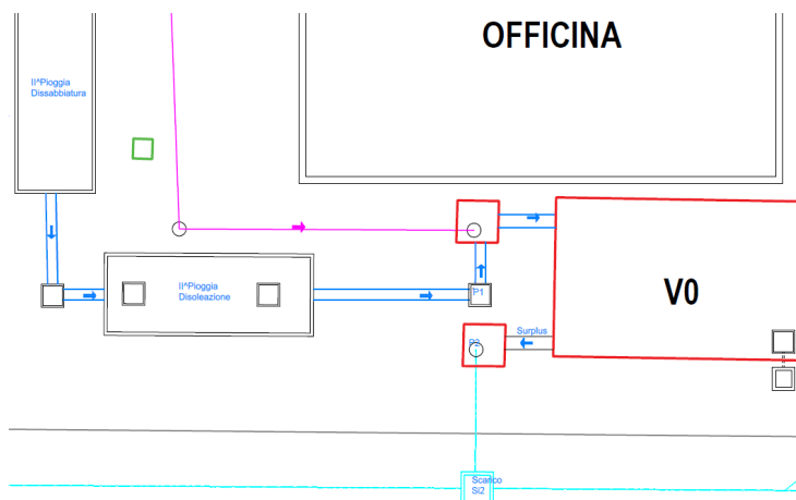
Figura 40: Ubicazione punti di scarico (situazione di progetto)
