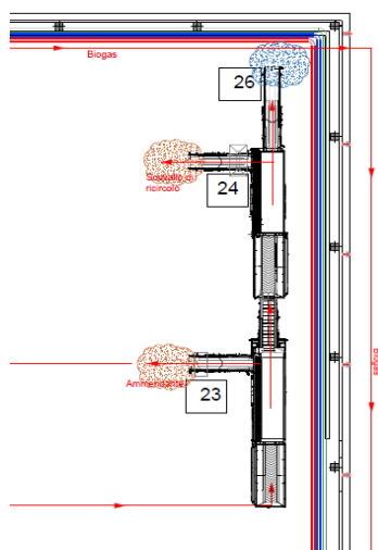
Figura 24: fase di vagliatura
