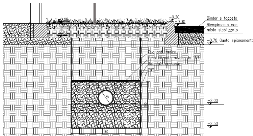
Figura 32: trincea drenante
