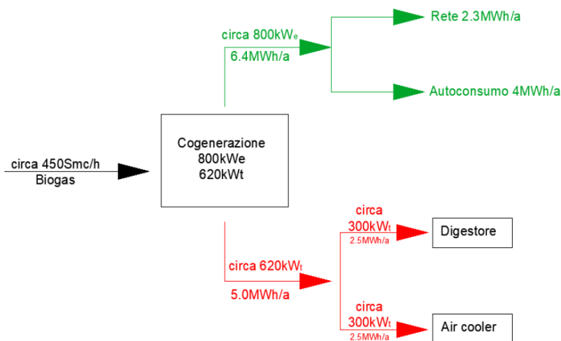
Figura 19: bilancio energetico del cogeneratore
