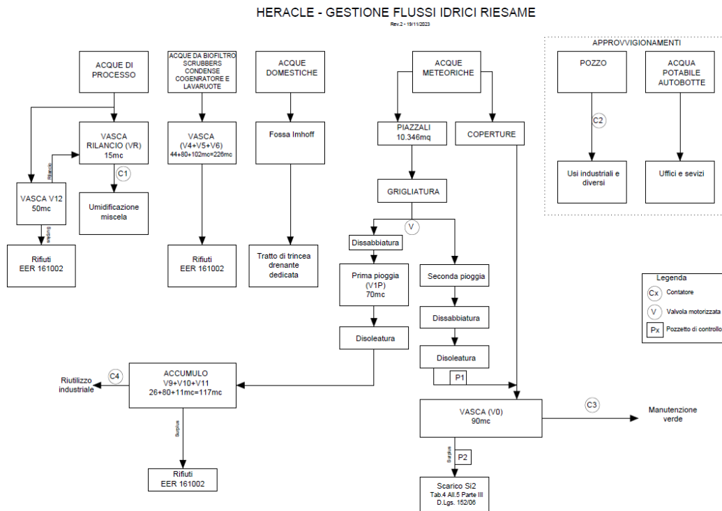
Figura 31: Schema di flusso gestione acque di stabilimento nella situazione di progetto
