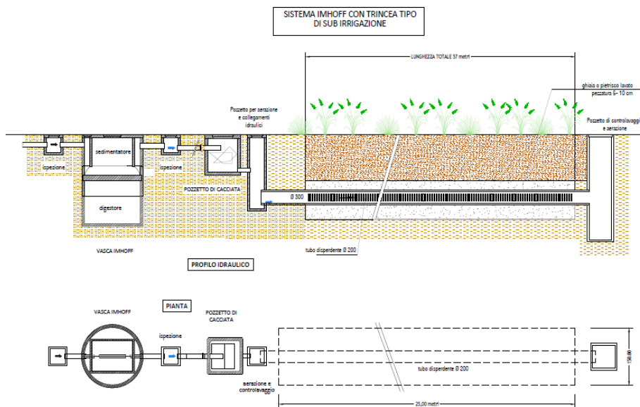
Figura 33: schema trattamento acque assimilate alle domestiche
