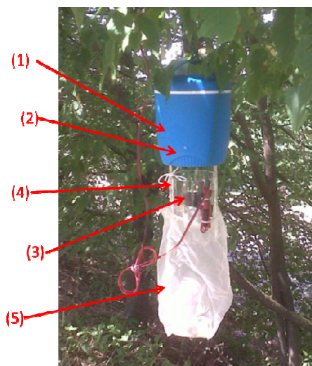
Figura 1: trappola tipo CDC modificata a CO 2 .
