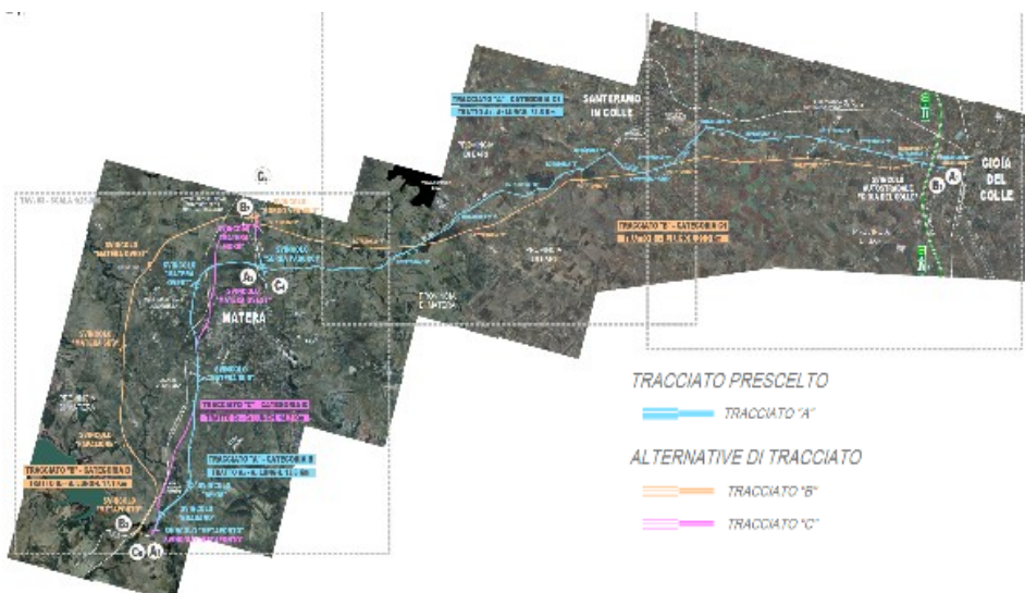
Corografia generale con indicazione delle tre alternative progettuali.
