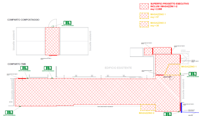
Fig.4 - stralcio estratto da Tav.9 bis rev.00 "Lay out nuove coperture" – Progetto oggetto di modifica
