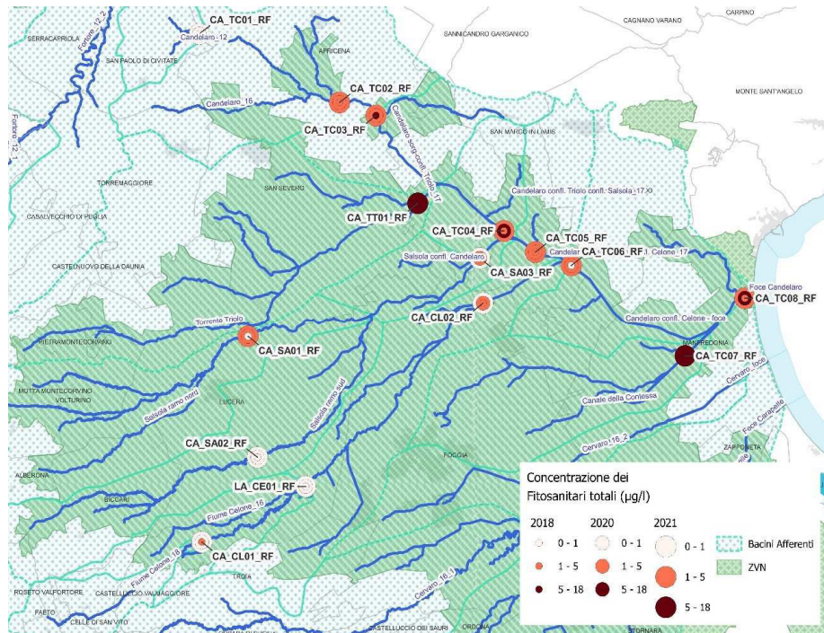
Figura 5.3 – Concentrazione di fitosanitari totali calcolati per le annualità di monitoraggio 2018, 2020 e 2021 per il contesto idrologico Candelaro.
