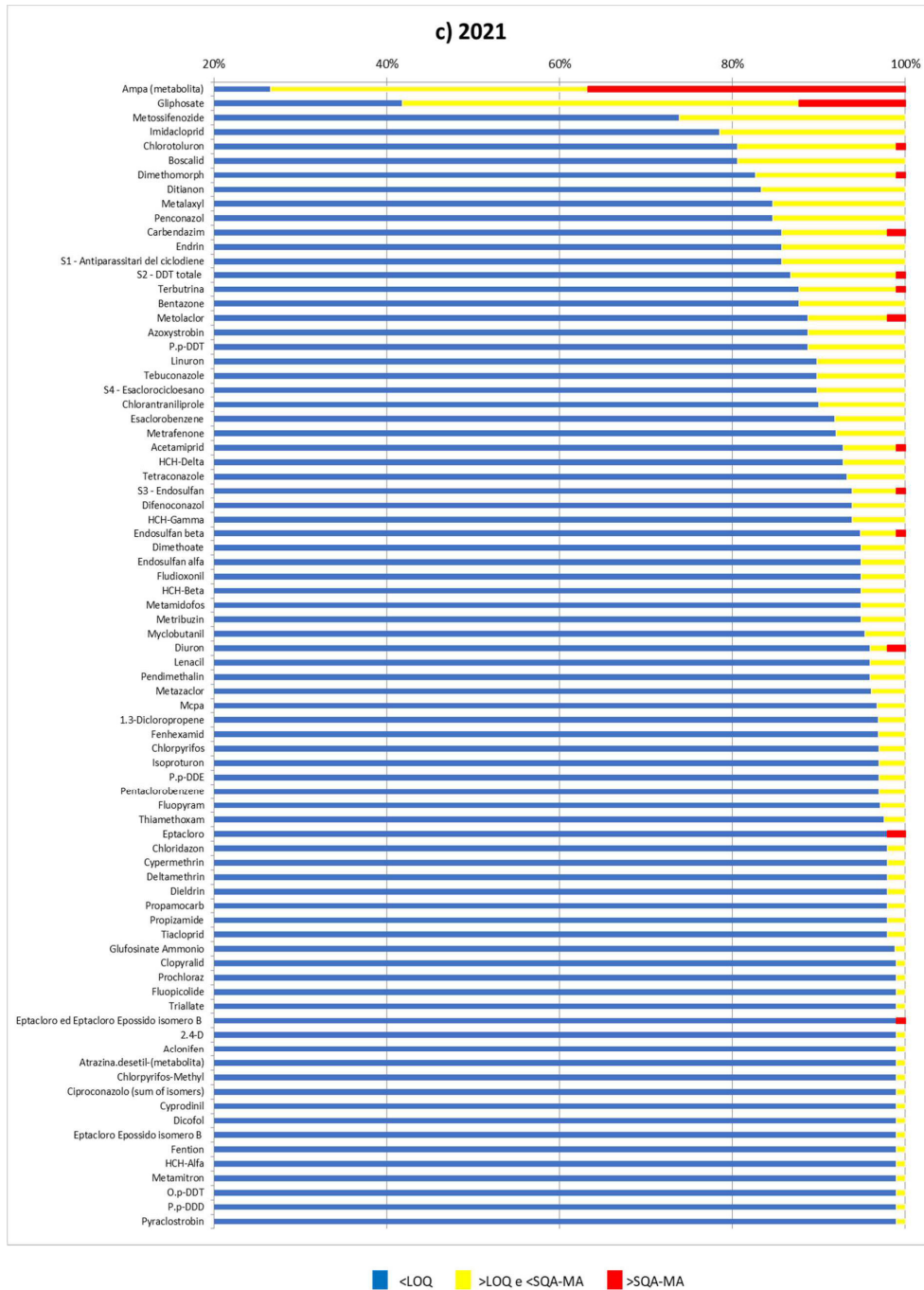
Figura 3.4 – Valori medi annui superiori al LOQ (in giallo) o superiori allo SQA-MA (in rosso) per le sostanze con almeno un ritrovamento nel 2018 (a), 2020 (b) e 2021 (c) (rispettivamente n. 57, n. 77 e n. 80 singole sostanze e sommatorie). Le sostanze sono riportate in ordine decrescente rispetto al numero di valori medi annui superiori al LOQ. Per una migliore visualizzazione dei dati si riporta uno stralcio dei grafici complessivo (valori sull’asse delle ascisse nell’intervallo 20-100%). Le valutazioni del 2018 sono relative all’unica campagna eseguita.
