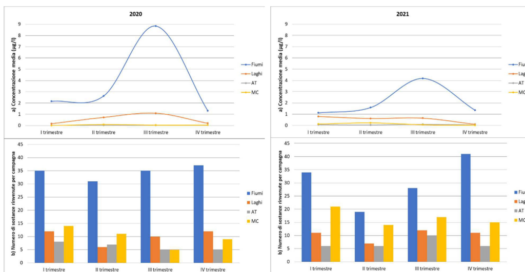
Figura 4.4 – Concentrazione media di fitosanitari totali (a) e numero di sostanze rinvenute (b) per campagna e per tipologia di corpo idrico (anni 2020 e 2021).
