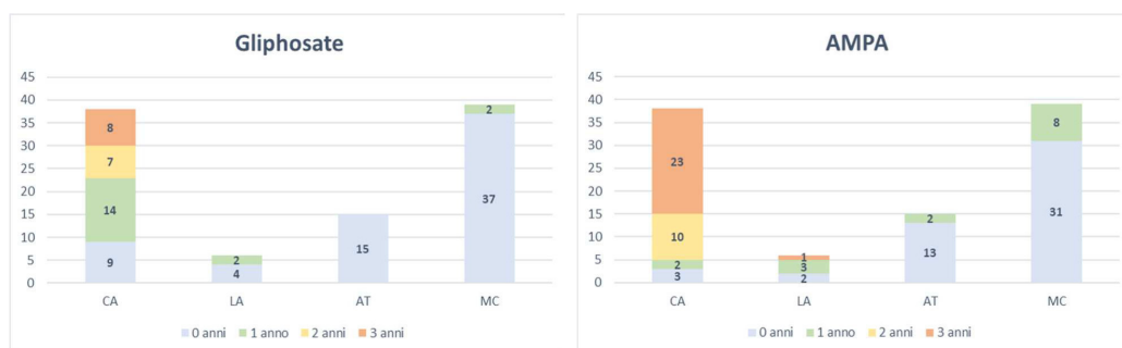
Figura 4.3 – Stazioni (n.) raggruppate per categoria e per numero di annualità con media > SQA-MA di Glyphosate e AMPA (anni 2018, 2020 e 2021).
