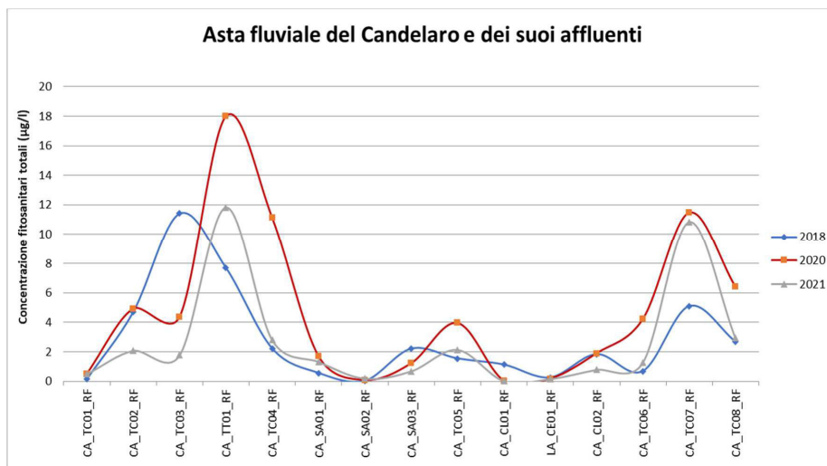
Figura 5.4 – Confronto tra i valori medi di concentrazione di fitosanitari totali calcolati per le annualità di monitoraggio 2018, 2020 e 2021 per il contesto idrologico Candelaro.
