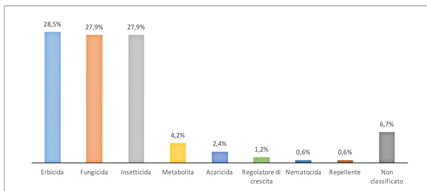
Figura 3.1 – Distribuzione percentuale delle sostanze determinate per categoria fitoiatrica di appartenenza.
