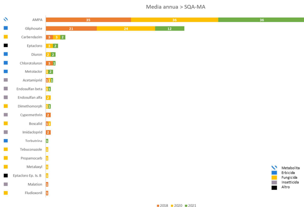
Figura 3.5 – Sostanze con superamenti dello SQA-MA (anni 2018, 2020 e 2021).
