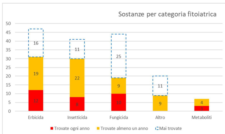
Figura 3.3 – Distribuzione percentuale delle sostanze trovate per categoria fitoiatrica rispetto alle annualità di monitoraggio.
