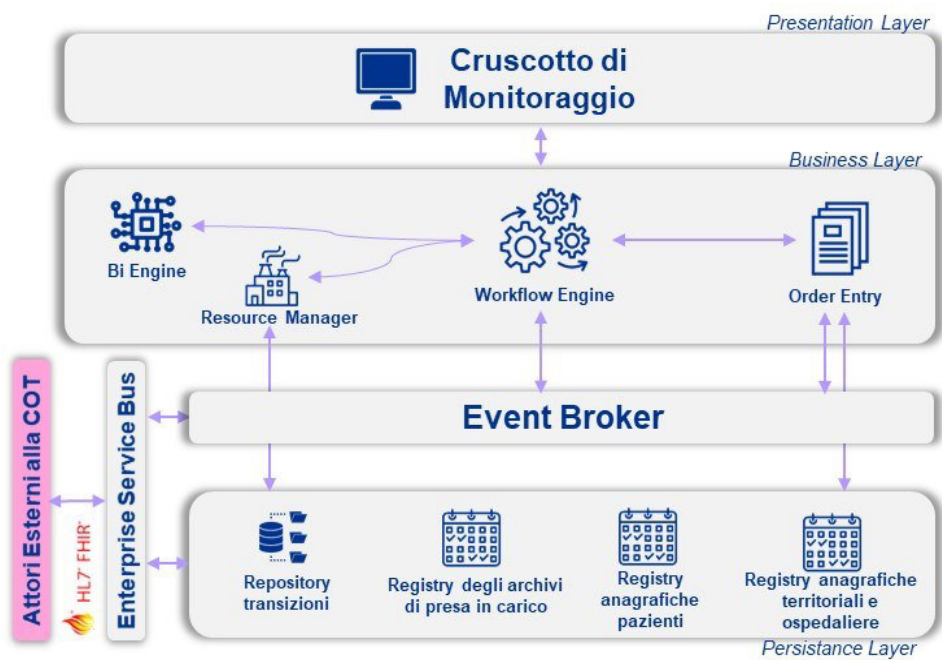
Figura 4 Architettura di riferimento COT
