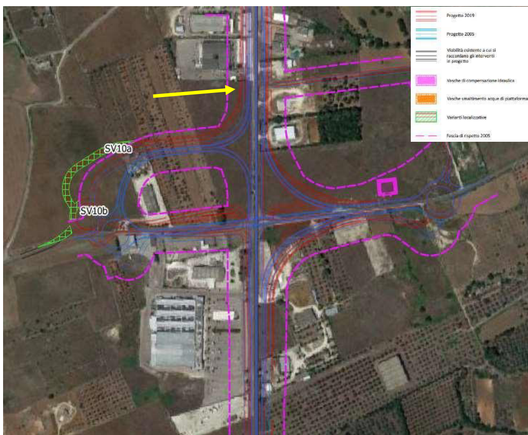
Figura 17: Svincolo 10 (Surano – Ruffano) con indicazione delle varianti localizzative SV10a e SV10b.
