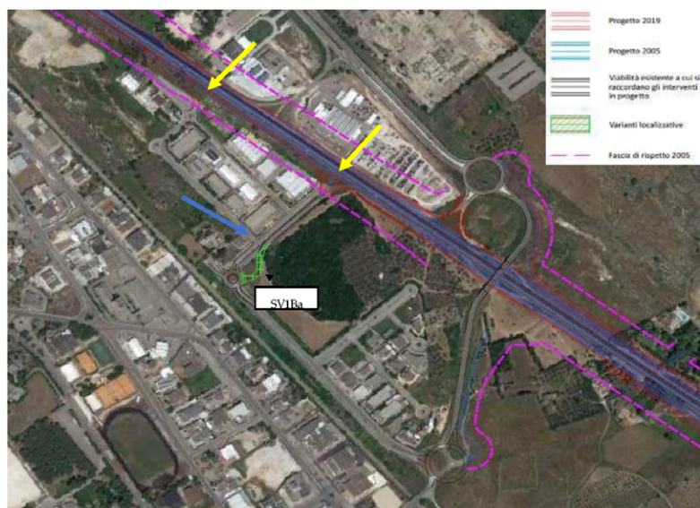
Figura 2 Svincolo 1b Zona industriale di Maglie con indicazione del tratto in variante localizzativa SV1a. Le frecce gialle indicano i nuovi raccordi da realizzare mentre la freccia blu indica la viabilità esistente oggetto di modifiche alla viabilità
