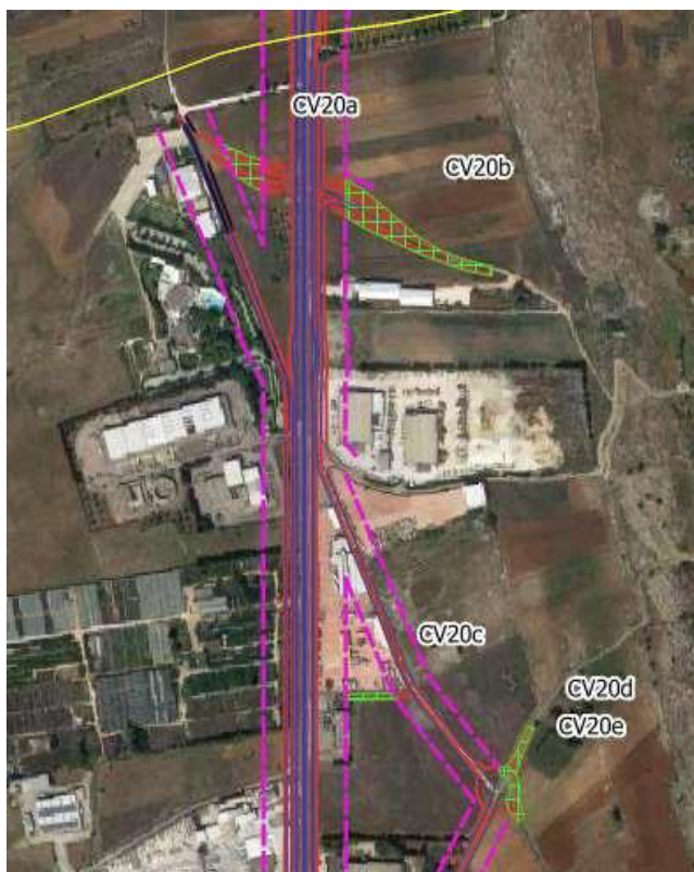
Figura 16 Scavalco 2 e complanare CV20 con indicazione delle varianti localizzative CV20a, CV20b, CV20c, CV20d e CV20e
