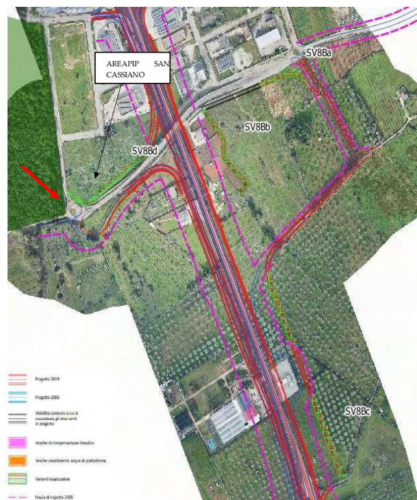
Figura 13 Svincolo 8b San Cassiano con indicazione delle varianti localizzative SV8Ba, SV8Bb, SV8Bc e SV8Bd.
