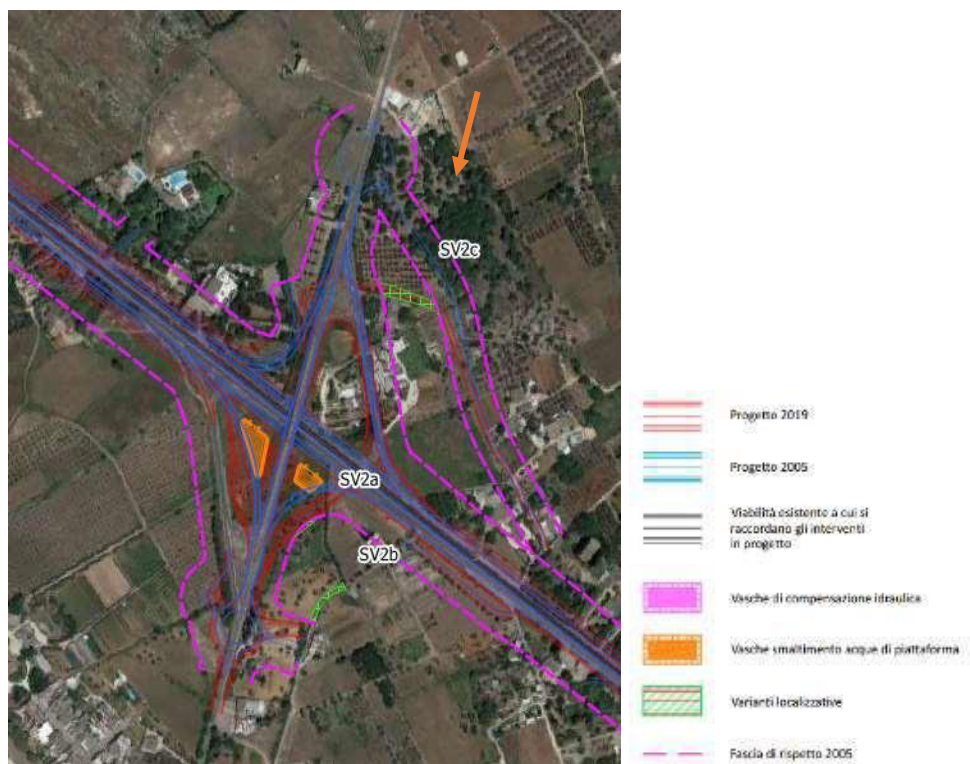
Figura 3 Svincolo 2 Corsi con indicazione delle varianti localizzative SV2a, SV2b e SV2c. Con la freccia arancione è indicato il bosco perimetrato da PPTR.
