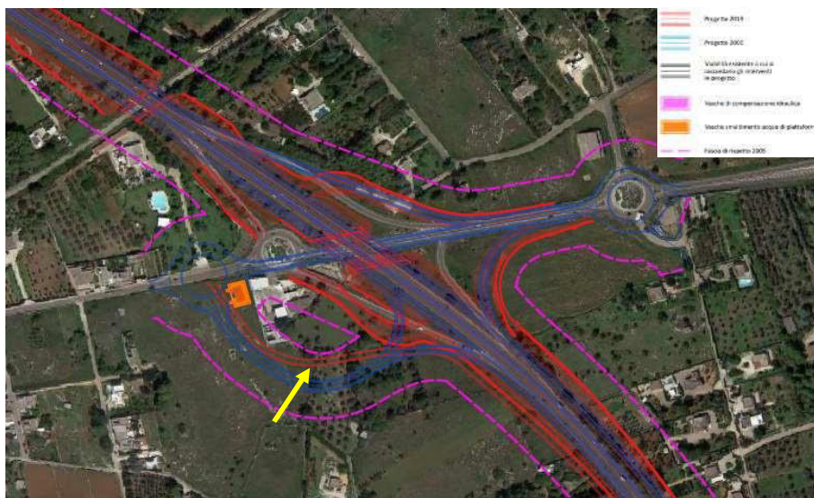
Figura 5 Maglie – Otranto. Con freccia gialla è indicata la complanare in variante non localizzativa
