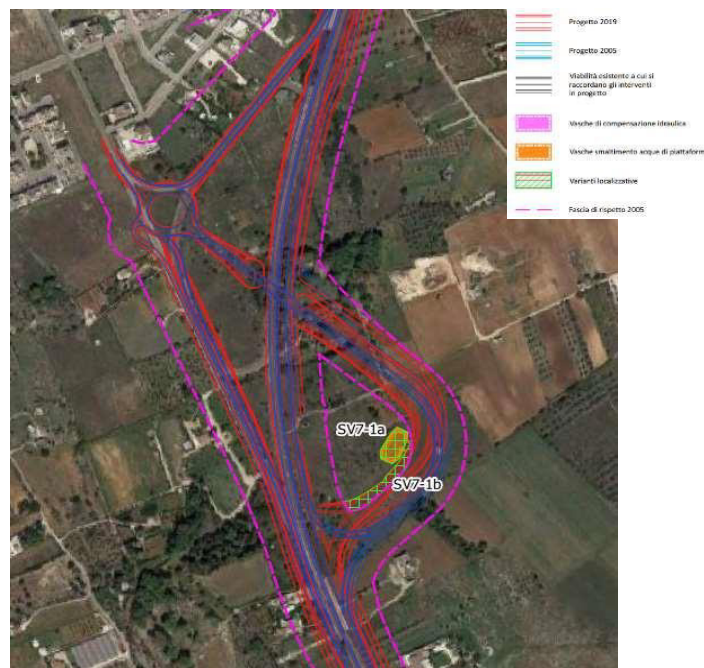
Figura 9 Svincolo 7 Scorrano Sud con indicazione delle varianti localizzative SV7a SV7b.
