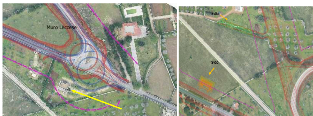
Figura 7 Lato est con indicazione del progetto revisionato in rosso e progetto approvato in blu; varianti localizzative svincolo 5.
