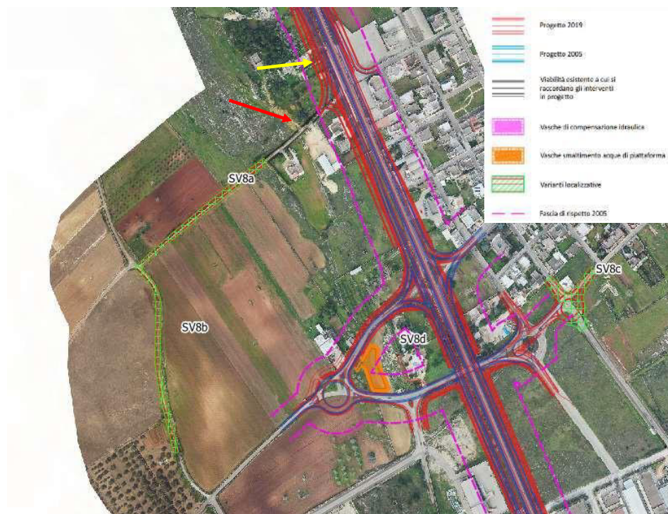
Figura 11 Complanare Botrugno con indicazione delle varianti localizzative SV8a, SV8b, SV8c e SV8d. La freccia gialla indica la variante alla quale la complanare si adegua.
