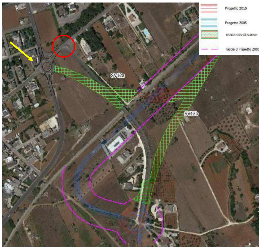
Figura 22: Svincolo 12 Montesano – Andrano con indicazione delle varianti localizzative SV12a e SV12b
