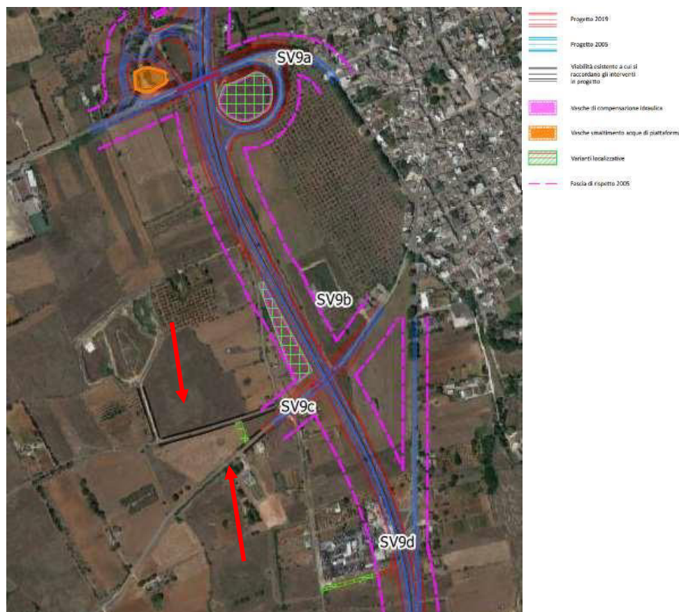
Figura 15 Svincolo 9b Nociglia Nord con indicazione delle varianti localizzative SV9a, SV9b, SV9c e SV9d
