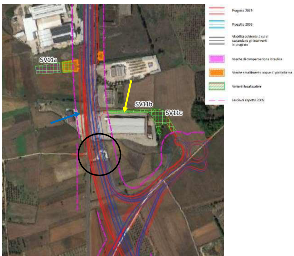
Figura 18: Svincolo 11 Montesano Nord con indicazione delle varianti localizzative SV11a, SV11b e SV11c.
