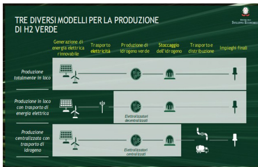
Figura 8 Produzione, trasporto e stoccaggio di H2 verde.
