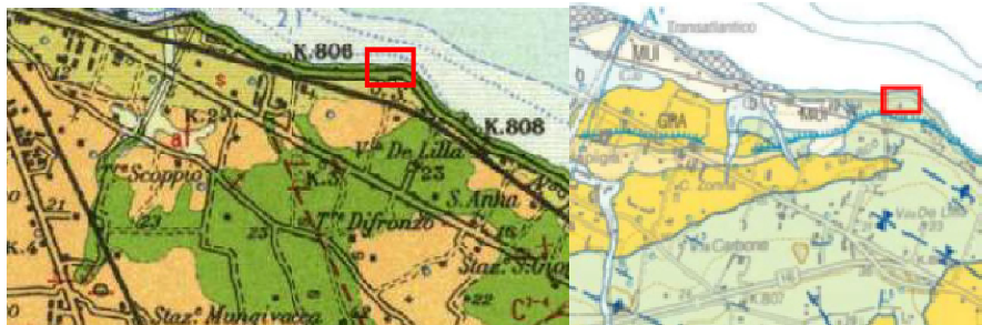
Stralcio della Carta Geologica d'Italia, (scala 1:100.000) Foglio 177 "Bari" Stralcio della Carta Geologica d'Italia, ed. CARG (scala 1:50.000) Foglio 438 "Bari"
