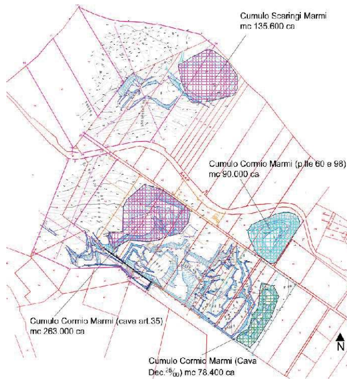
Fig. 11_Estratto Tav. 6 (Integrazioni febbraio 2020-Volumetria cumuli)
