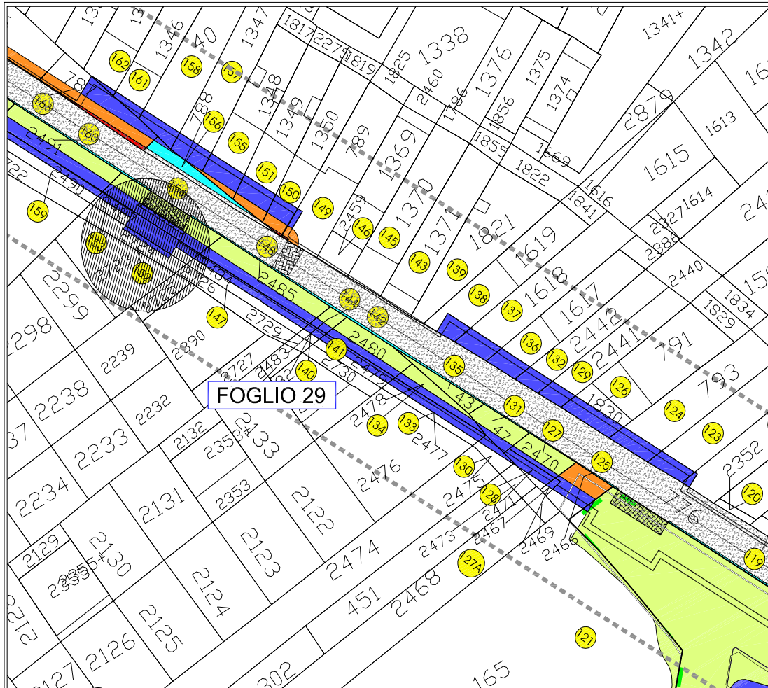
Stralzo del Piano Particellare Scala 1 : 1000
