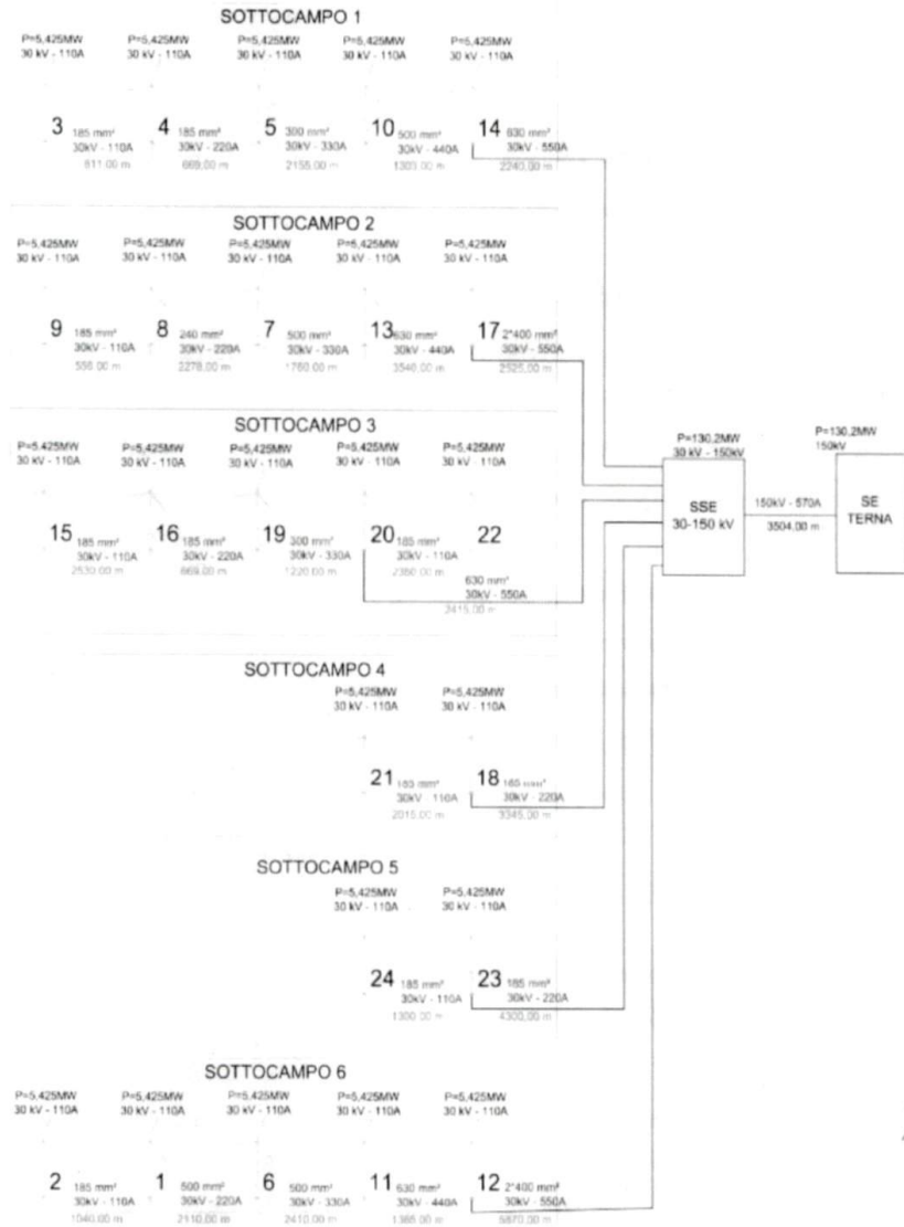
Figura 3: schema di collegamento estrapolato dall'elaborato "R.9" (RELAZIONE SPECIALISTICA OPERE ELETTRICHE)
