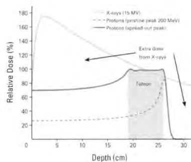
Figura 2 - Picco di Bragg
