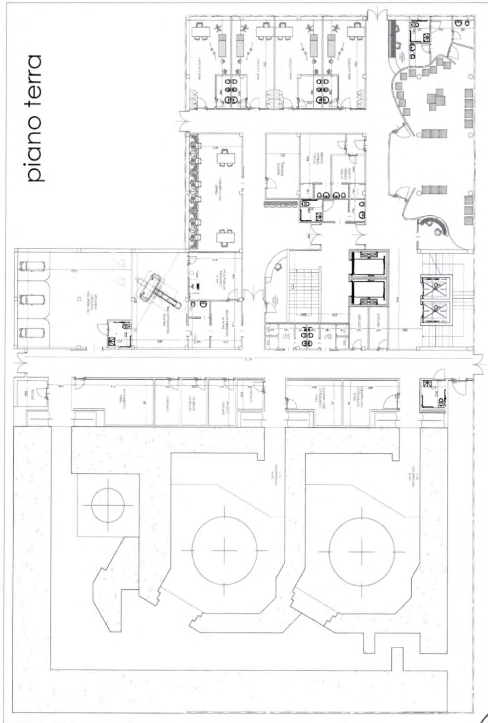
Fig. 15 - ipotesi di distribuzione planimetrica del piano terra
